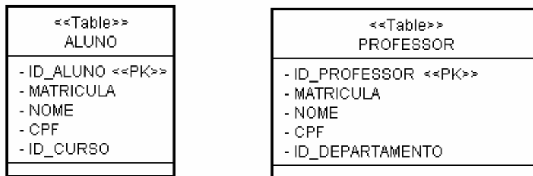
Figura 18 - Tabela por Classe Concreta
