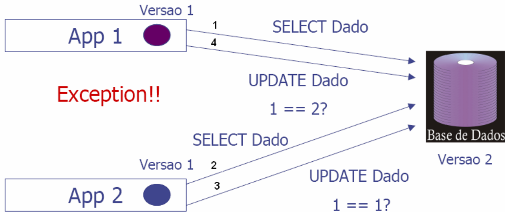
Figura 23 - Locking Otimista: Abodargem com Version Number
